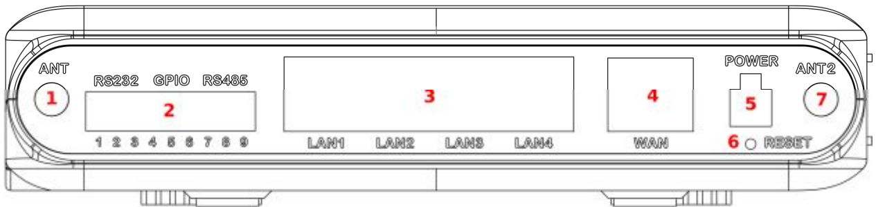
Рис. 3.1. Вид сзади
