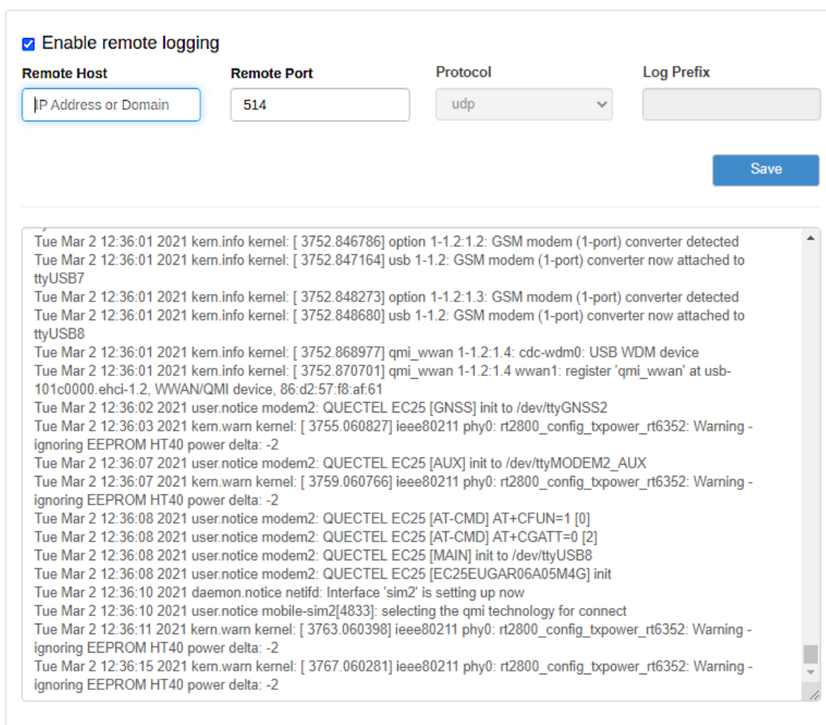
Рис. 57. Вкладка Tools, раздел System Log
