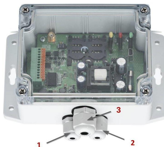
Рис. 17. Обозначение гермовводов.
